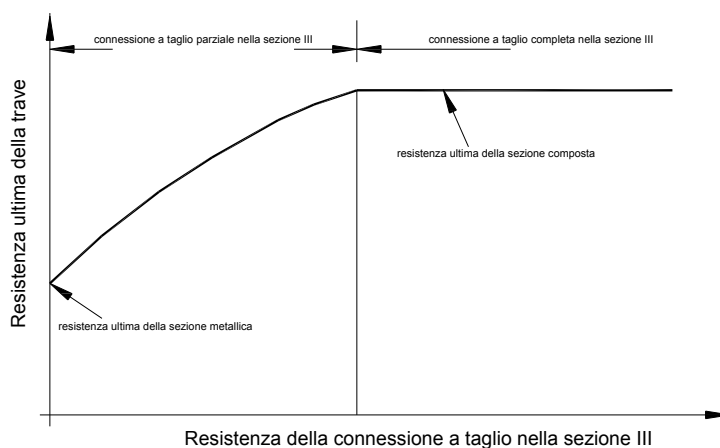
Figura C4.3.6 – Legame tra resistenza della trave e resistenza della connessione
